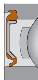
RSR Einlippendichtung
